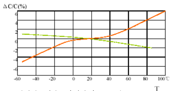
电容变化率与温度关系(在 1kHz 时)
